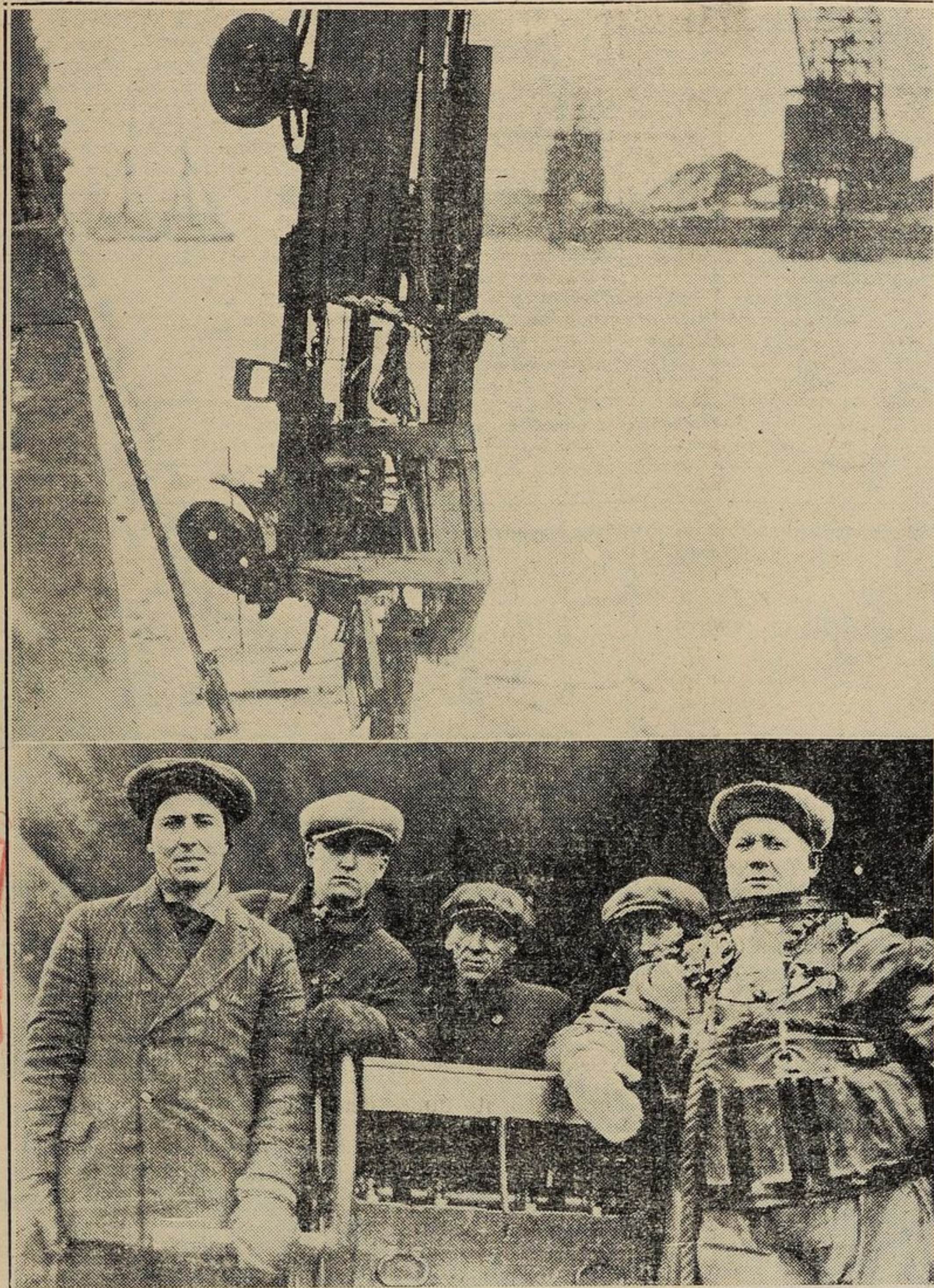
In alto: Un camion sollevato dall'acqua mediante una gru meccanica. Sotto lo scafandro, che discese a 45 piedi sotto l'acqua per attaccare le catene attorno al camion.
